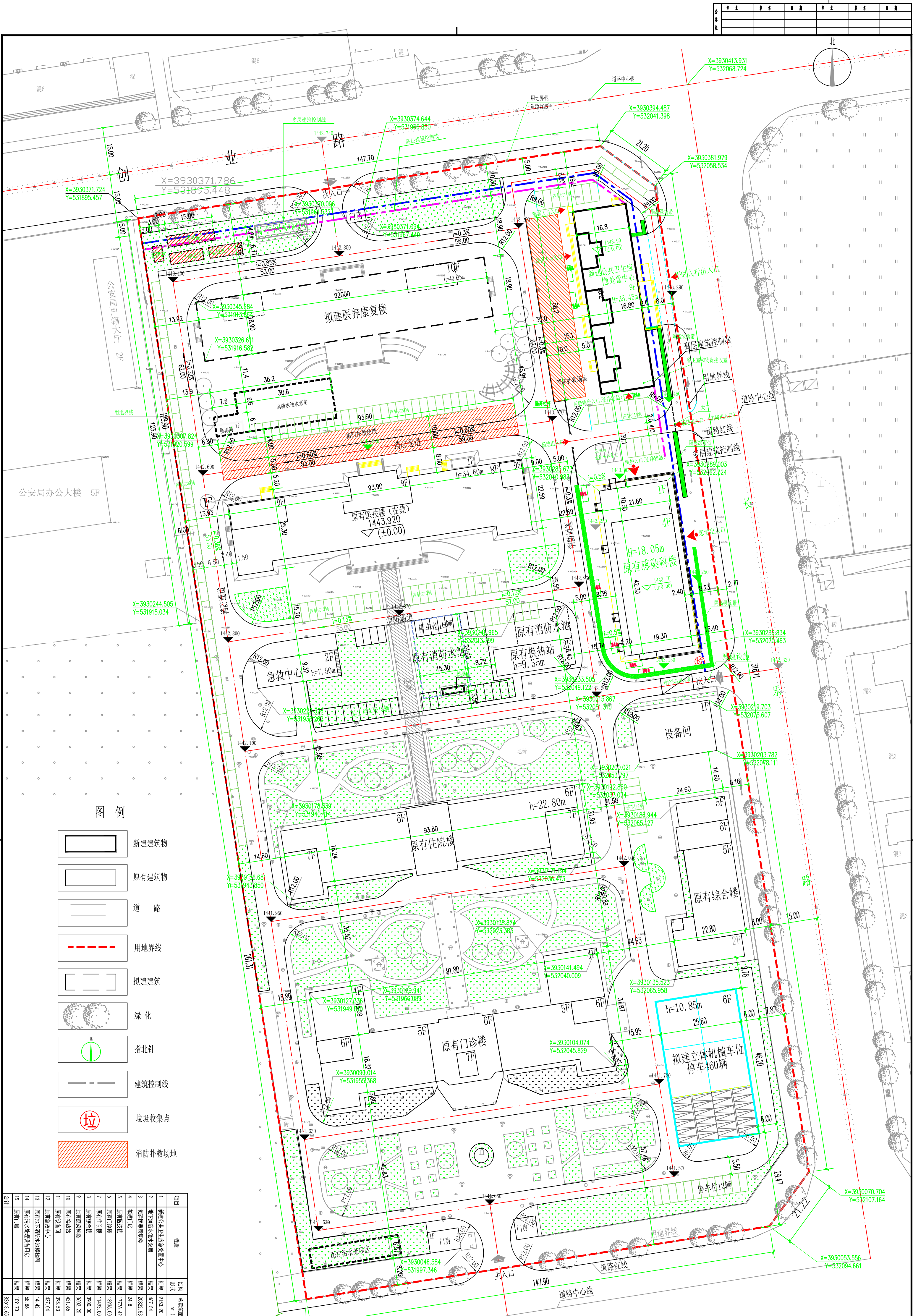
总平面布置图 1:500
